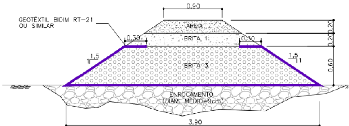
Figura 1: Seção típica – Dreno de fundo tipo 4. Fonte CSN Mineração, 2021 a , 2021 b
